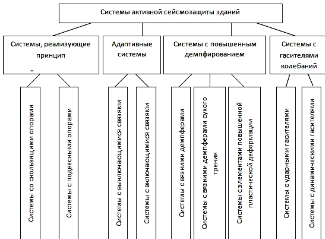
2.11-расм. Фаол сейсмик ҳимоя системаси классификацияси
