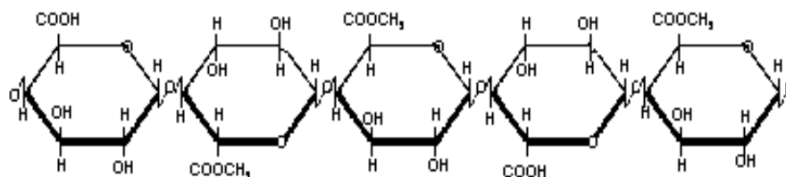
пектин
