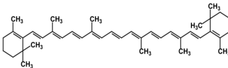
β-каротин
