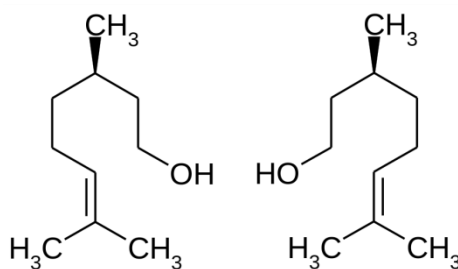
Цитронеллол
