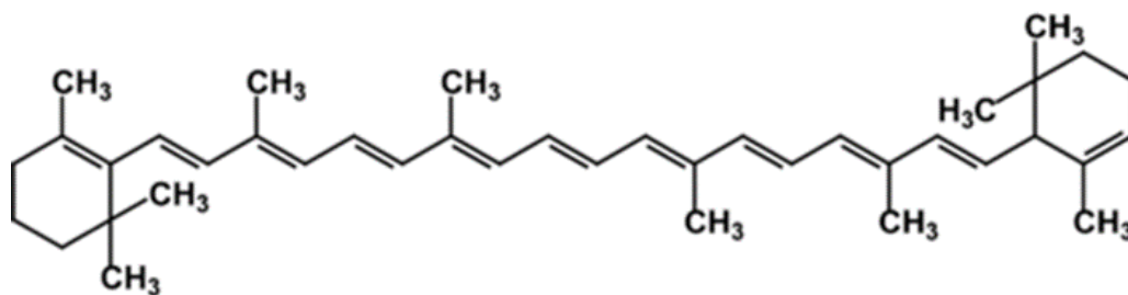
каротин
