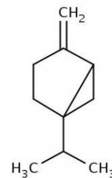
Сабинен
