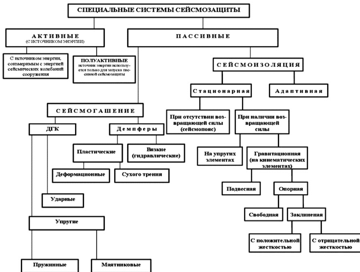
2.10-расм. Сеймик ҳимоя тизимларининг классификацияси ва уларнинг ишлаш тамойиллари
