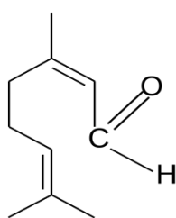
Цитраль
