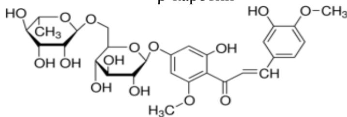
Гесперидин
