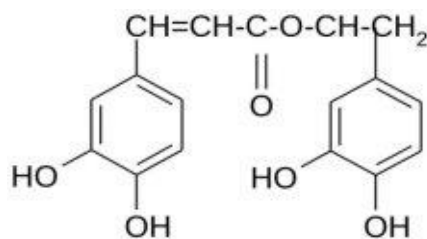
Хлороген кислота
