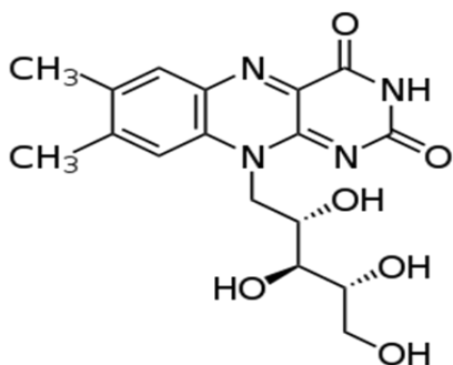
Рибофлавин
