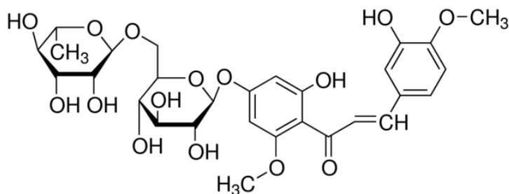
Гесперидин
