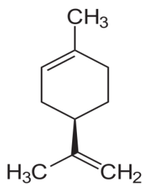
Лимонен
