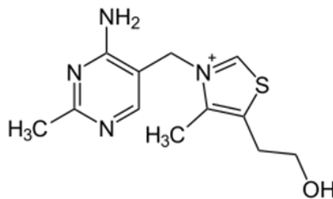
тиамин
