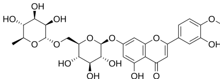
Диосмин
