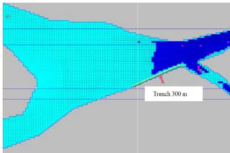
4-расм. Пионер хандак мавжуд бўлганда оқим ҳаракати.
