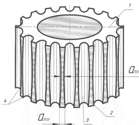
Рис.1. Питающий цилиндр прядильного устройства
