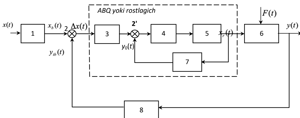
1-rasm. Bir o'lchamli oddiy ABT funksional sxemasi.
