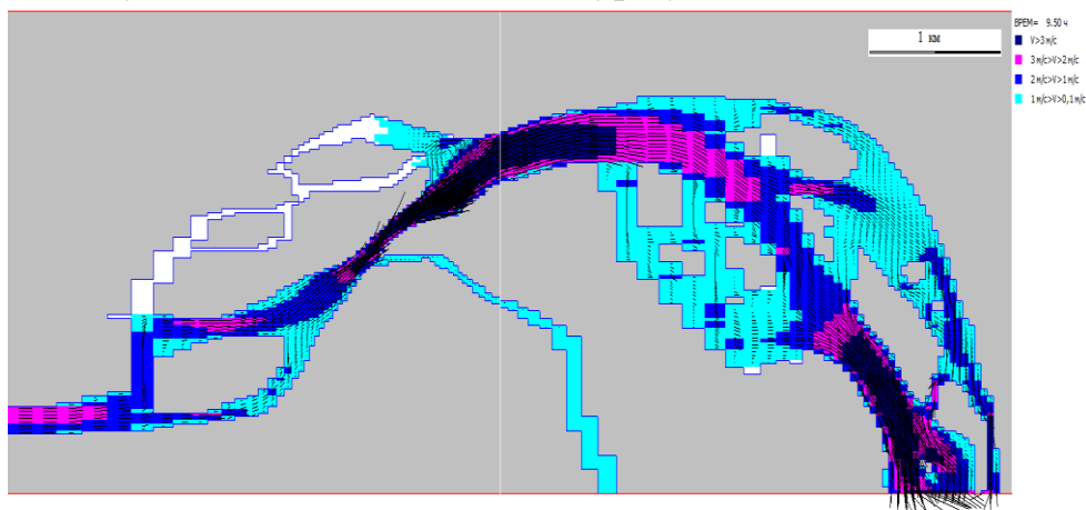
3-расм. Амударёнинг Аму-Бухоро машина каналига тўғонсиз сув олиш бош иншооти соҳасидаги оқимнинг ҳаракати меженъ даврида ҳеч қандай муҳандислик тадбирлари ўтказилмаган ҳолат учун оқим ҳаракати ( Q_k=100 m^3/c , n=0,021 )
