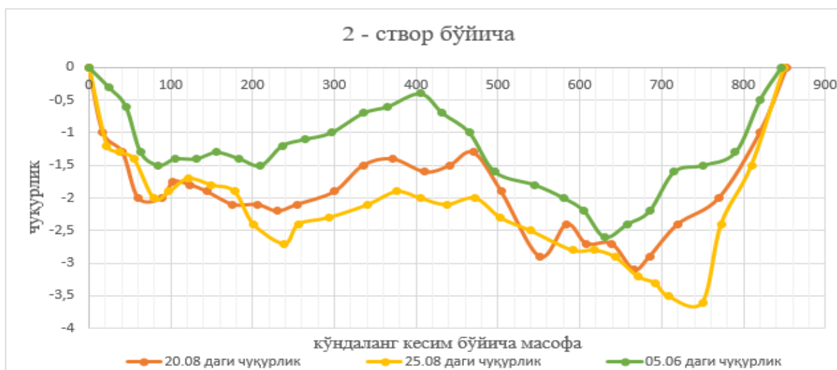
1-расм. АБМК тўғонсиз сув олиш ҳудудида қўйи қисми Амударё ўзани туби кўндаланг кесим динамикаси.
