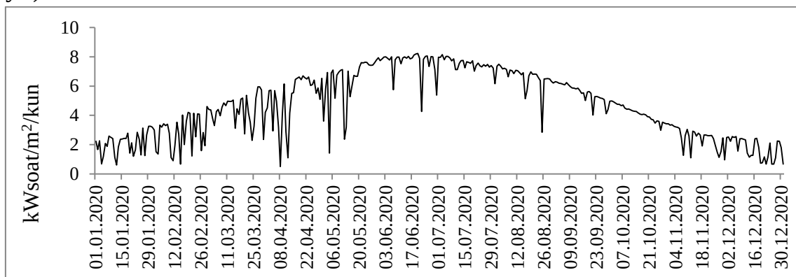
2-rasm. Buxoro viloyatida quyosh batareyalaridan olinadigan kunlik solishtirma energiya ko'rsatkichlari (2020 yil).
