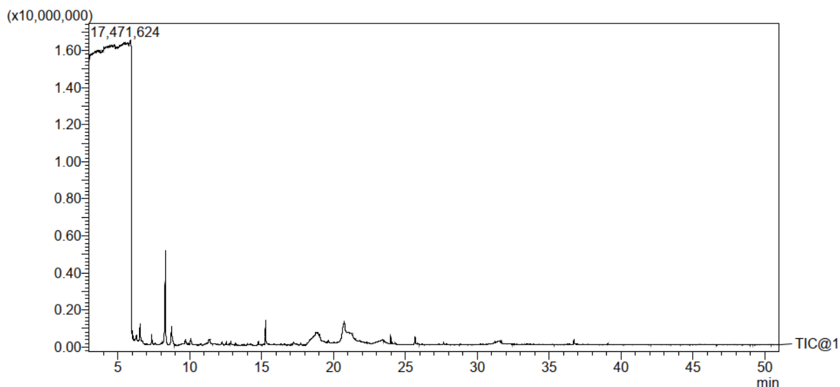
Рисунок ИМС-хроматограмма
