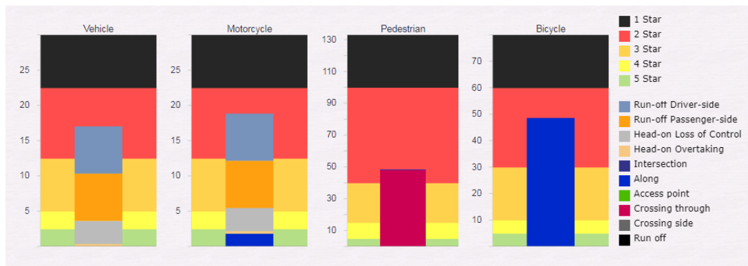
Рис. 5. Показатели риска для участников дорожного движения на автомобильной дороге 4P21.
