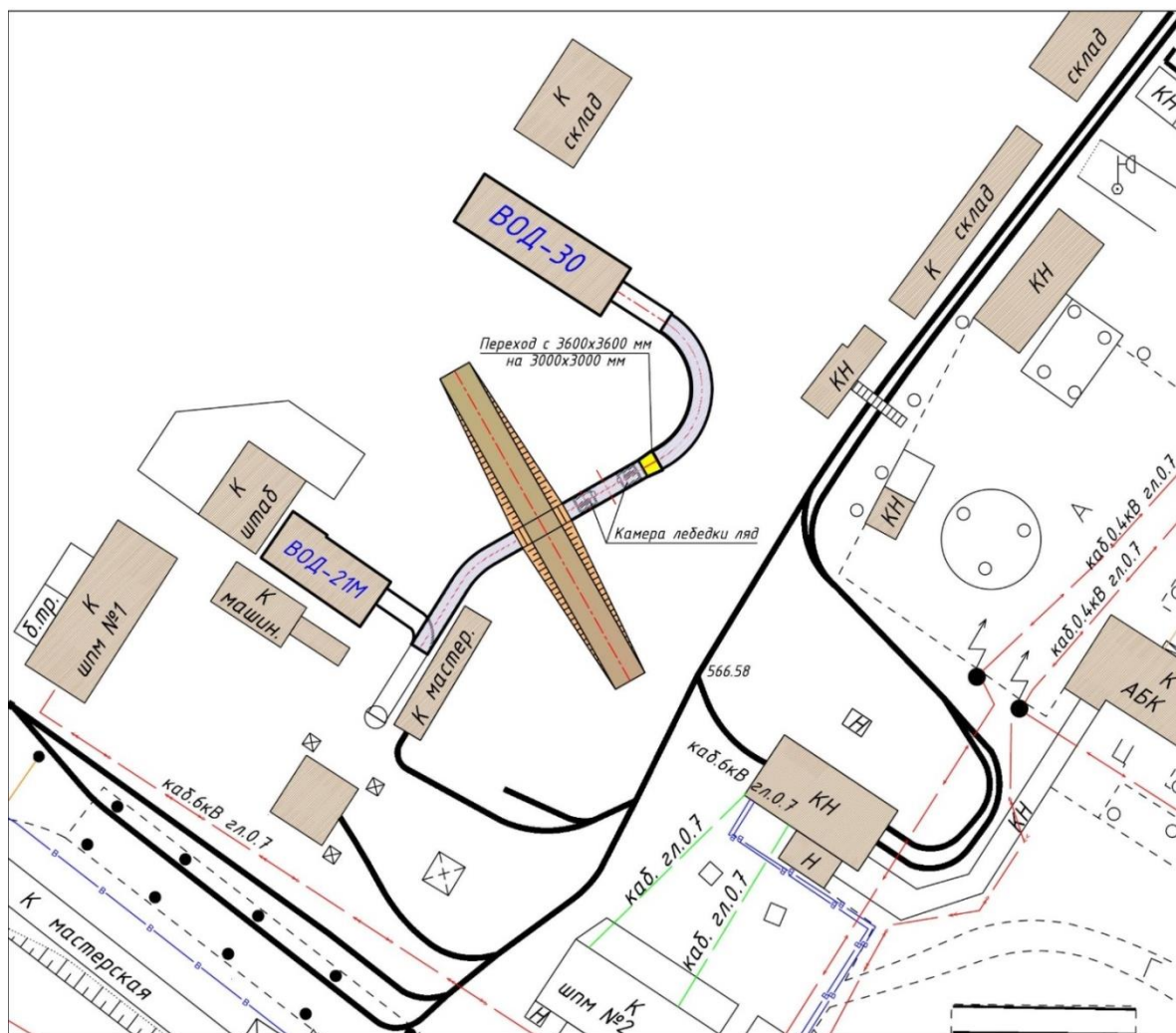
Рис. 1. «Присоединение вентиляционного канала вентилятора ВОД-30 к вентиляционному каналу вентилятора ВОД-21 шахты «М»»
